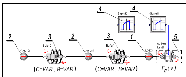
Фиг. 2. 1-блок-локомотив, 2-блок-вагони, 3-буферен блок, 4-сигнал-генераторни блокове, 4-блок-силово натоварване
