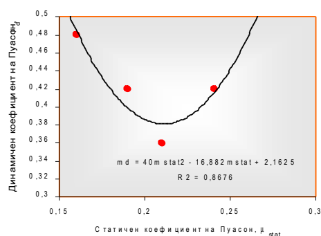
Фиг. 3. Връзка между статичния ( \mu_{stat} ) и динамичния ( \mu_d ) коефициенти на Пуасон
