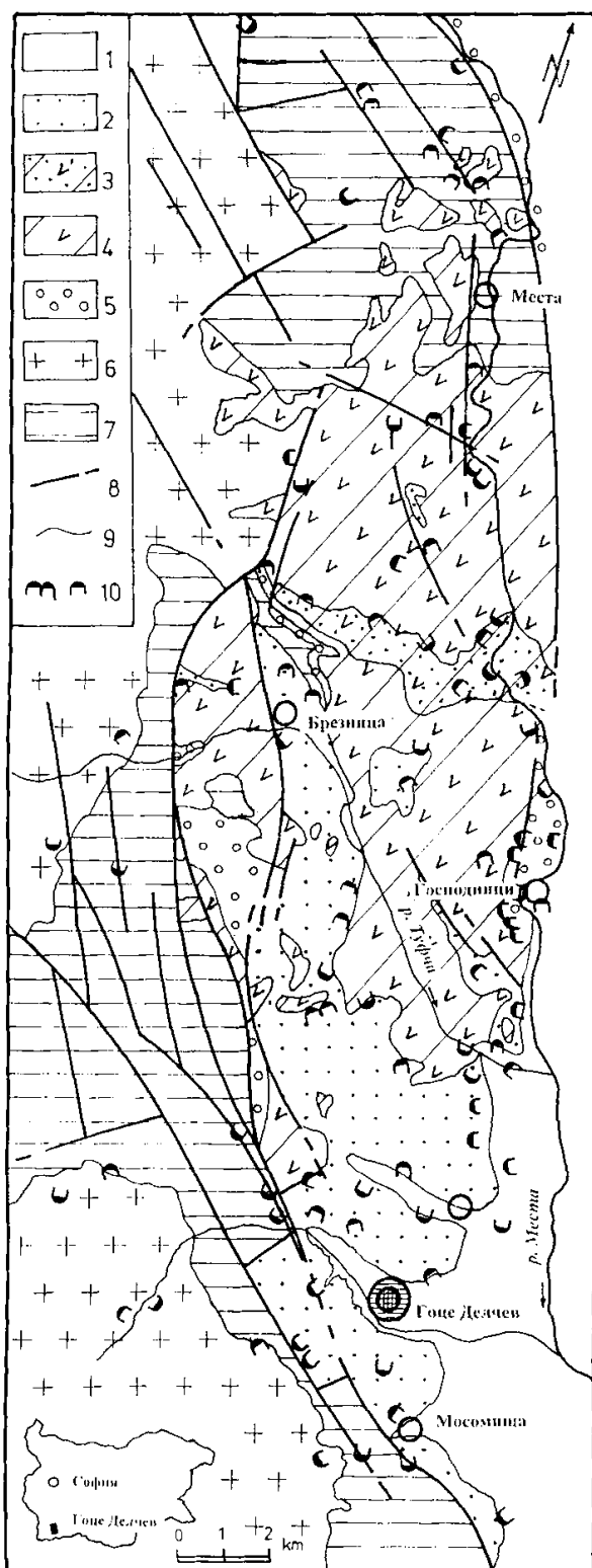
Фиг. 1. Геоложка схема и карта на разпространението на свлачищата в западната част на Местенския грабен, северно от гр. Гоце Делчев. Геоложките данни са по Геоложката карта М 1:100 000 и допълнения по материали на автора
