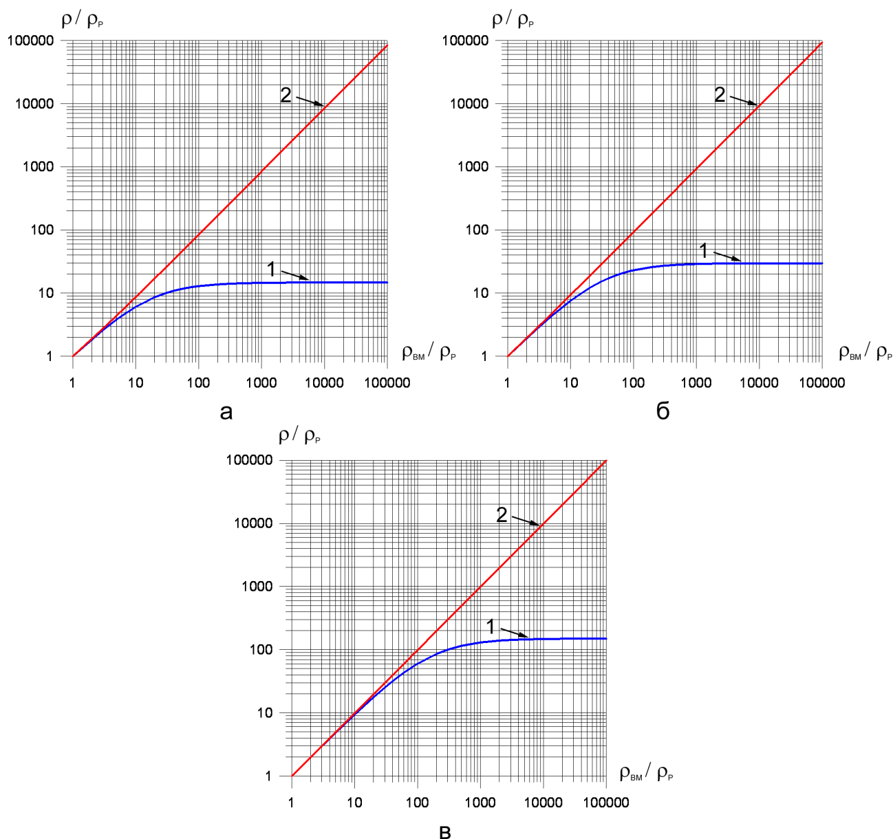
Фиг. 5. Графики на разпределението на специфичните електрически съпротивления за двуконпонентна среда при модел, приложим за прожилкова (графики 1) и впръсната (графики 2) минерализация при съдържание на електропроводящата компонента съответно 10% (а), 5% (б) и 1% (в)
