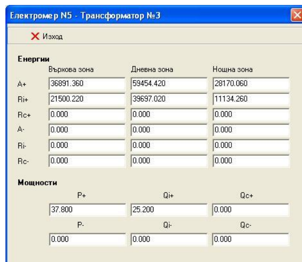
Фиг. 2. Екранна форма за извеждане на моментни показания на електромер или контролна точка
