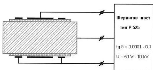
Фиг. 2. Опитна постановка за измерване на коефициента на диелектричните загуби \text{tg}\delta
