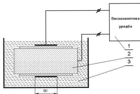
Фиг. 1. Опитна постанова за изпитване на пробивно електрическо напрежение
