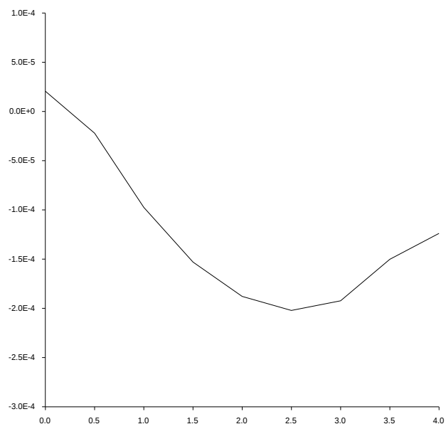
Фиг. 2. Напрежения \sigma_y по сечение „19-27“
