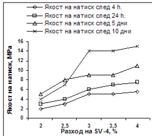
Фиг. 5. Зависимост между разхода на свързващо вещество SV-4 и якостта на натиск на брикетите
