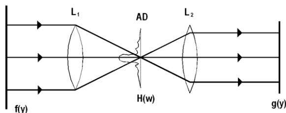
Фиг. 1. Оптична система с ограничаваща апертура
