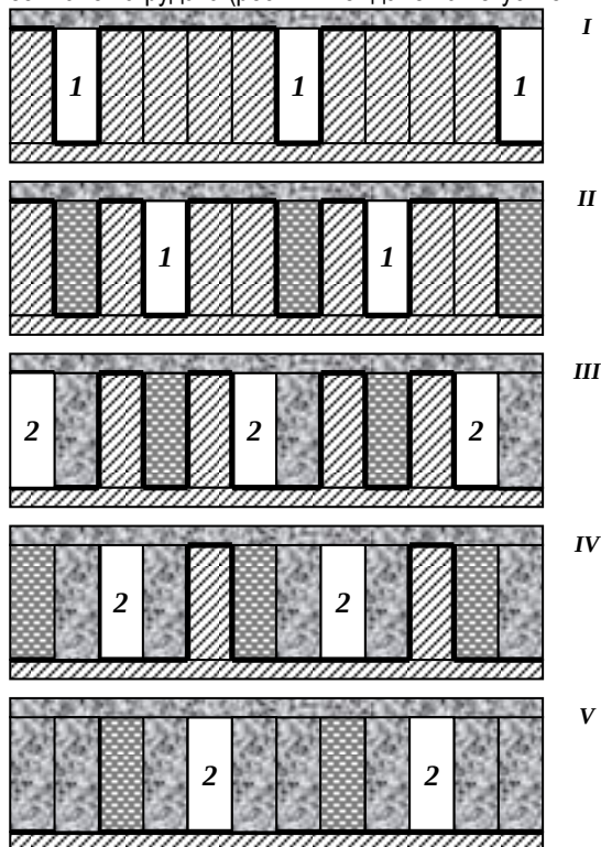
Фиг. 3. Камерно-цементова система на разработване – вариант едновременно изземване на 1/5 част от запасите на блока; I, II, ..., V – последователност на изземване на камерите; 1 – първични камери; 2 – вторични камери
