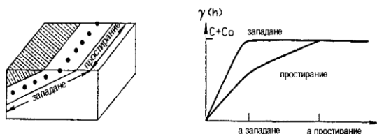
ГЕОМЕТРИЧНА АНИЗОТРОПИЯ
