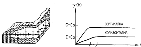
ЗОНАЛНА АНИЗОТРОПИЯ
