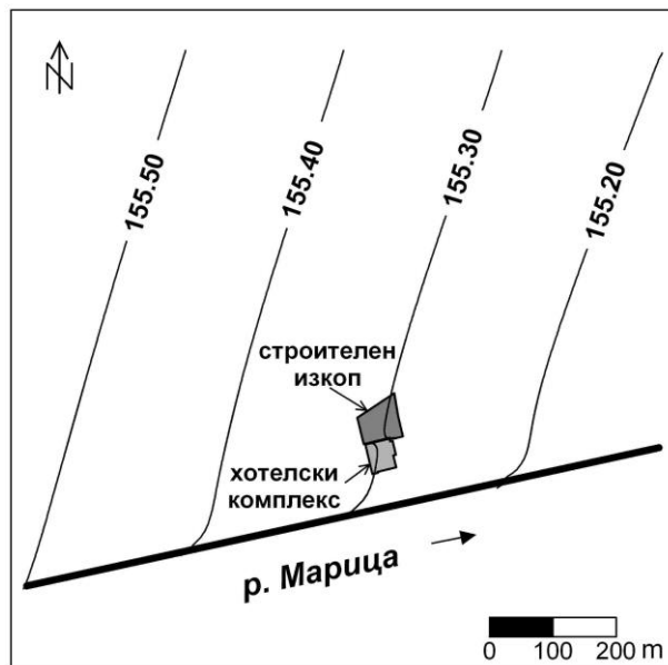
Фиг. 2. Структура на ненарушеното филтрационното поле
