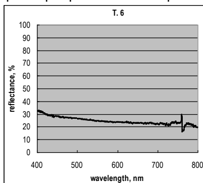
Фиг. 6. Спектрална характеристика на доломит
