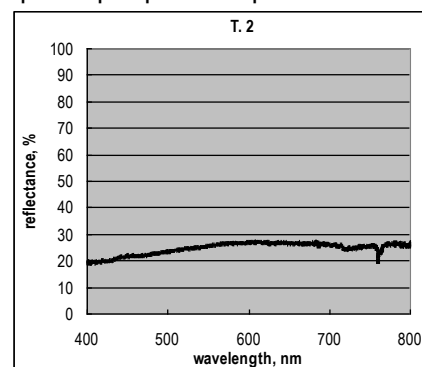
Фиг. 2 Спектрална характеристика на биотитов гнайс
