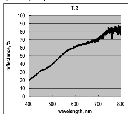
Фиг. 3. Спектрална характеристика на гнайс
