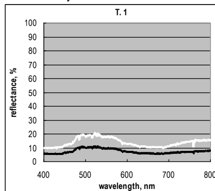
Фиг. 1 Спектрални характеристики на гранити
