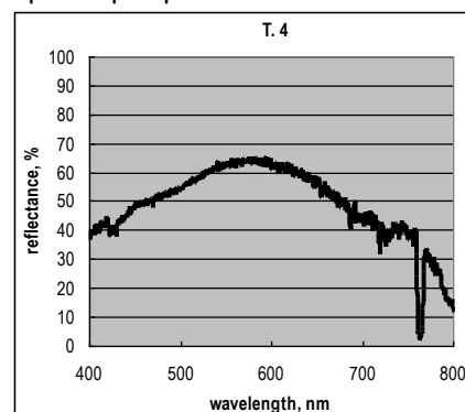
Фиг. 4. Спектрална характеристика на брекчоконгломерати
