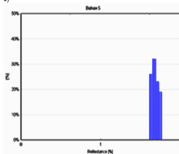
Фиг. 2. Рефлектограми на показателя на отражение на витринита. а) за проба 1; б) за проба 10; в) за проба 5
