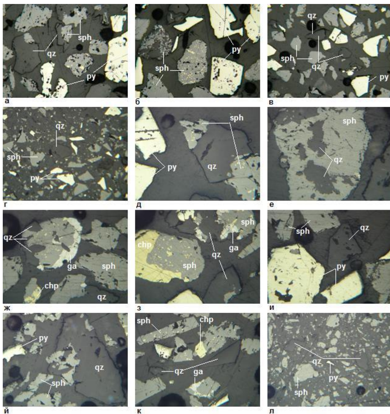
Фиг. 1. Микроскопски фотографии на препарати от колективен цинково-пиритен концентрат и технологичен цинков концентрат (отразена светлина, успоредни николи – N II, размер на видното поле: а-в – 1.04 mm, г-л – 0.53 mm; sph – сфалерит; py – пирит; chp – халкопирит; ga – галенит; qz – кварц): а) срастъци на кварц със сфалерит – в горната и в лявата част на кадъра (около тях – фрагменти от сфалерит и пирит, обр. №9); б) сфалерит, силно кородиран от финозърнести кварцови агрегати – в лявата част на кадъра (вдясно – сфалерит с фини и емулсионни включения от халкопирит, пирит със зонално разположени включения от кварц и други нерудни минерали, обр. №9); в) две свободни зърна от кварц – в горната половина на кадъра (около тях – фрагменти и идиоморфни индивиди пирит и частици от сфалерит, обр. №10); г) ксеноморфно зърно от кварц – в централната част на кадъра (около него – фрагменти от сфалерит и пирит, обр. №11); д) срастък на кварц със сфалерит (вляво – фрагменти от пирит, обр. №18); е) сфалерит с включения от кварцови агрегати (вдясно – фрагмент от кварцово зърно, обр. №18); ж) сфалерит-галенитов агрегат, кородиран от кварц (в долната половина на кадъра вляво – срастък на сфалерит с халкопирит, вдясно – срастък на сфалерит с кварц, обр. №18); з) срастък на кварц със сфалерит, галенит и халкопирит – в горния десен ъгъл (вляво – агрегат от халкопирит и сфалерит с емулсионни включения от халкопирит; кварцов индивид с включения от сфалерит – в долния десен ъгъл, обр. №18); и) свободно зърно от кварц – в централната част на кадъра (в горния ляв ъгъл – фрагменти от сфалерит; в долния ляв ъгъл – пирит с ксеноморфни включения от кварц и сулфиди; вдясно – сфалерит с финозърнести кварцови агрегати, обр. №18); й) срастък на кварц с триъгълни очертания със сфалерит (вляво – единична пиритова частица и фрагменти от сфалерит, обр. №19); к) ксеноморфно кварцово зърно – вляво и кварцов фрагмент с триъгълни очертания – вдясно (в горния десен ъгъл – срастък на сфалерит с халкопирит; в долната част на кадъра – срастък на сфалерит с галенит, обр. №19); л) ксеноморфни зърна от кварц (около тях – фрагменти от сфалерит и единична частица пирит, обр. №20)
