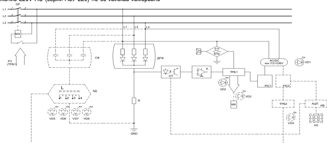
Фиг. 1 Блокова схема на апарат за общомрежова защита от тока на утечка с непрекъснат контрол на изоляционното съпротивление в IT мрежи
