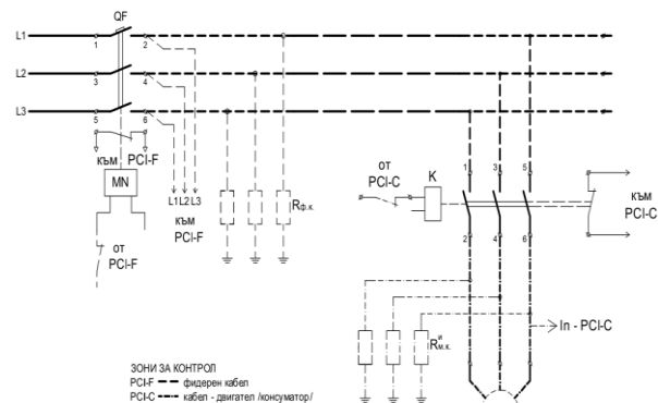
Фиг.3. Блокова схема на апарат за защита от токови утечки с предварителен контрол на изолационно съпротивление
