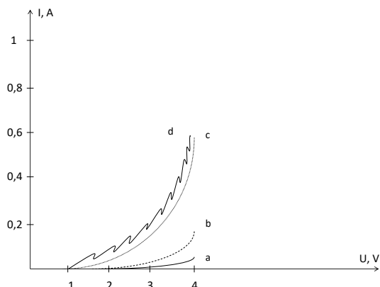
Фиг. 3: Волт-амперни характеристики на етапите на производство на молекулярен светодиод
