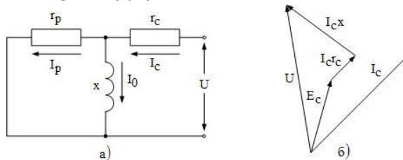
Фиг.1 Заместваща схема (а) и векторна диаграма (б) на асинхронен двигател
