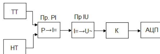
Фиг.1 Структурната схема на канал за измерване на мощност.
