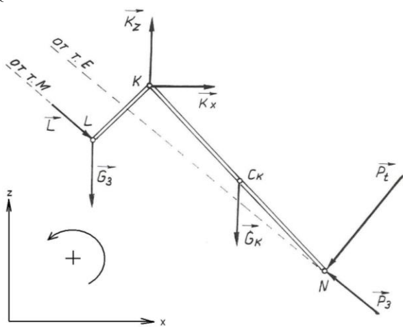
Фиг. 4. Сили действащи на кофата на багера
