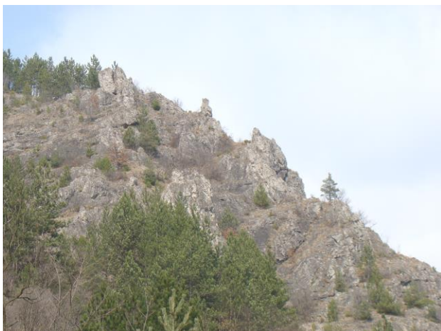
Фиг. 5. Скални пирамиди с височина до 5-6 m от ансамбъла на група 4, разположена в десния склон на Гарванов дол
