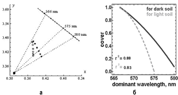
Фиг. 4. Координати на цветността на грах върху тъмна • и светла ○ почва при различно растително покритие (а) и регресионни зависимости между проективното покритие на грах и доминиращата дължина на вълната на смесения клас при тъмна ---- и светла - - - почва (б)
