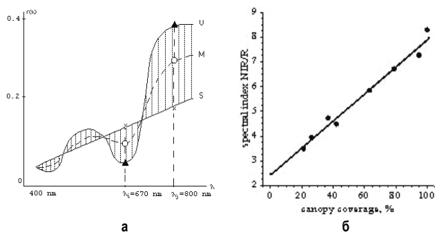
Фиг. 1. Спектрални отражателни характеристики на гола почва S (x), плътна растителна покривка V (▲) и смесен клас "почва-растителност" M (○) (а) и зависимост на вегетационния индекс NIR/R от растителното покритие на ечемик върху сива горска почва (б)
