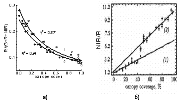
Фиг. 2. Зависимост на вегетационния индекс R/(G+R+NIR) (а) от растителното покритие на пролетен ечемик върху сива горска почва (1) и чернозем (2) и на вегетационния индекс NIR/R (б) на грах върху алувиално-ливадна почва за две фенофази
