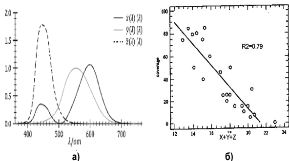
Фиг. 3. Стандартни CIE цветови функции (а) и зависимост на проективното покритие на пролетен ечемик върху сива горска почва в периода братене-вретене и сумата на цветовете координати – (б)
