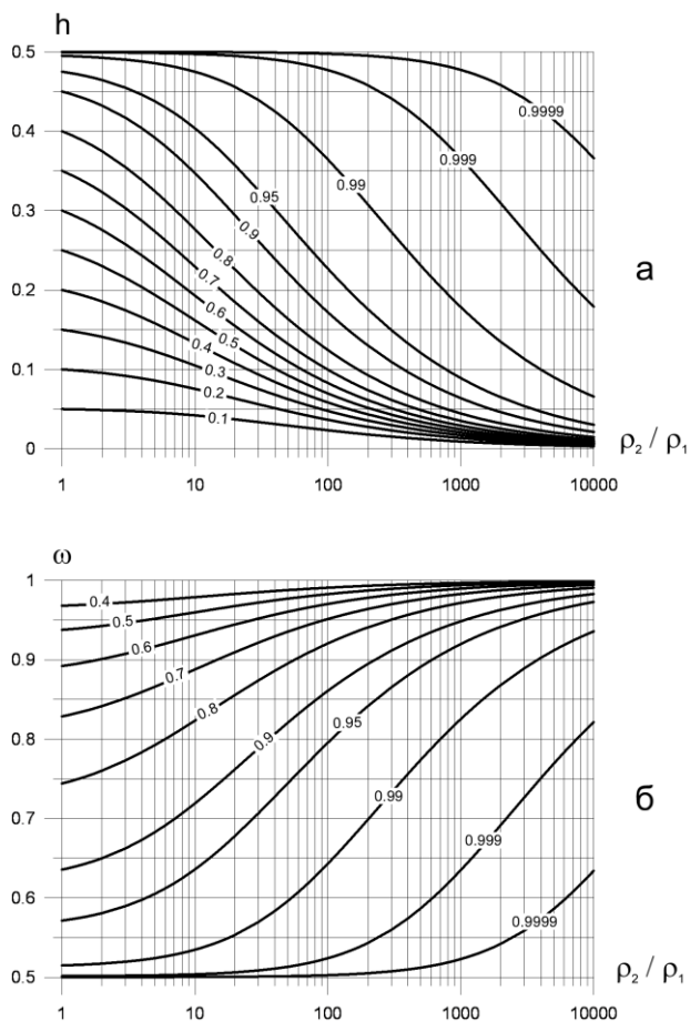
Фиг. 8. Графики на зависимостите \lambda_{\max} = f(h, a, \rho_2/\rho_1) (а) и респективно \lambda_{\max} = f(\omega, a, \rho_2/\rho_1) (б) при тип на контрастност \rho_2 > \rho_1 . Параметър на графиките е дължината a на ръба на квадратната основа на включението – паралелепипед (пластина)
