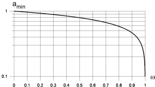
Фиг. 4. Връзка между минималната възможна дължина на ръба a на квадратната основа на включението под формата на паралелепипед (пластина) и специфичния обем \omega на вместващата компонента с електрично съпротивление \rho_1
