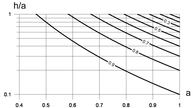
Фиг. 5. Взаимовръзка между отношението h/a и дължината a на ръба на квадратната основа на включението – паралелепипед (пластина). Параметър на графиките е специфичния обем \omega вместващата компонента с електрично съпротивление \rho_1
