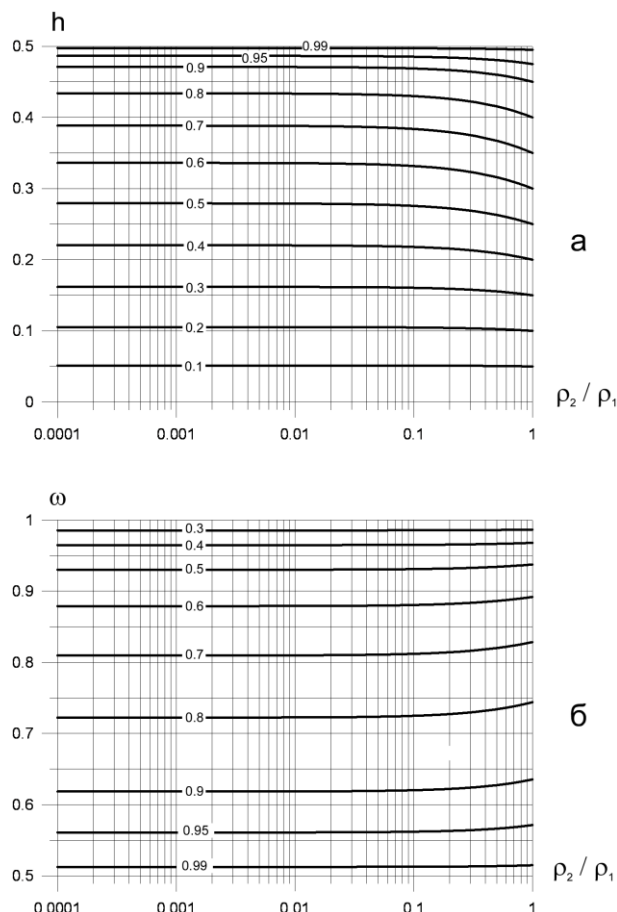
Фиг. 9. Графики на зависимостите \lambda_{\max} = f(h, a, \rho_2/\rho_1) (а) и респективно \lambda_{\max} = f(\omega, a, \rho_2/\rho_1) (б) при тип на контрастност \rho_2 < \rho_1 . Параметър на графиките е дължината a на ръба на квадратната основа на включението – паралелепипед (пластина)
