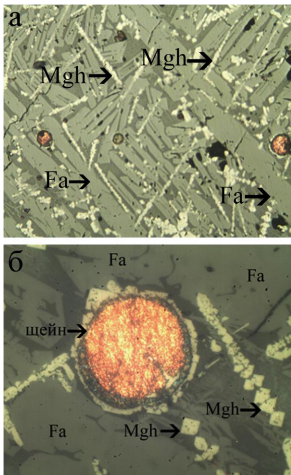
Фиг. 4. Микроскопски снимки на изследваните образци в отразена светлина: а – фаялит (Fa) с тъмносив цвят и магнезит (Mgh) със светлосив цвят в проба 16, размер на видното поле 850 μm; б – сулфидни (щейнови) агрегати, фаялит (Fa) и магнезит (Mgh) в проба 16, размер на видното поле 425 μm.
