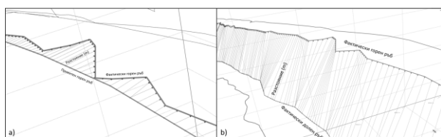
Фиг. 7. Пространствен анализ на фактически и проектни ръбове на рудника: а). оценка на разрушение в бермата между проектен и постигнат горен ръб; б). Измерване на разстояние между възлите на постигнат долен и горен ръб на рудника за определяне на ъгъла на единичен откос.
