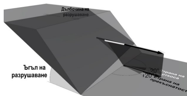
Фиг. 2 Дълбочина и ъгъл на разрушаване за плоско плъзгане. С бяла стрелка е показан векторът, описващ страната на откоса, а с тъмна – векторът, описващ страната на прекъснатостта. Показан е ъгъл 20° в едната и другата страна от страната на откоса.
