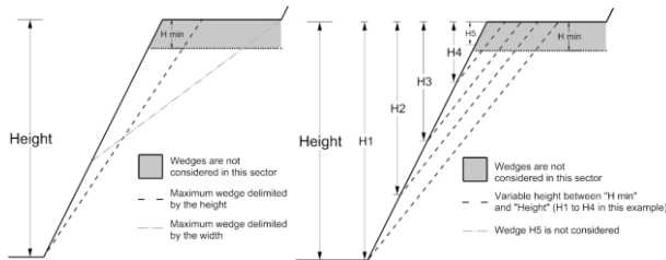
Фиг. 3 Генерирани разрушавания при фиксирана височина (вляво) и варираща – вдясно. И в двата случая могат да бъдат изключени разрушения с височина по-малка от минимално приетата (от User’s Manual KATS 2018).
