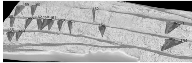
Фиг. 5. Ортофото модел на клинове в сектор 7 на рудника. Пространствените характеристики на прекъснатостите изграждащи всеки клин са измерени и използване при изчисление на коефициента на устойчивост. Номерацията на всеки клин е както в Таблица 5.
