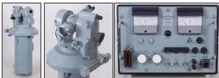
Фигура 26. Жиротеодолит Gi-B2
