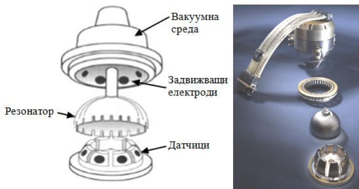
Фигура 19. Конструктивни елементи в устройството на HRG- схема и изображение: https://airandspace.si.edu
