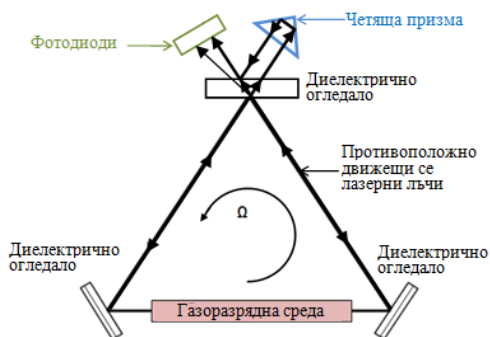
Фигура 12. Схема на лазерен жироскоп с основните конструктивни елементи
