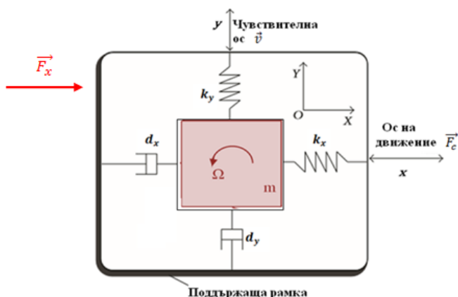
Фигура 17. Схема на CVG- чувствителен елемент с маса m и еластично окачване: \Omega - ъглова скорост на въртене на жироскопа, ос x и y - съответно ос на движение и чувствителна ос, коефициенти на еластичност ( k_x, k_y ) и коефициентът на затихване ( d_x, d_y ).
