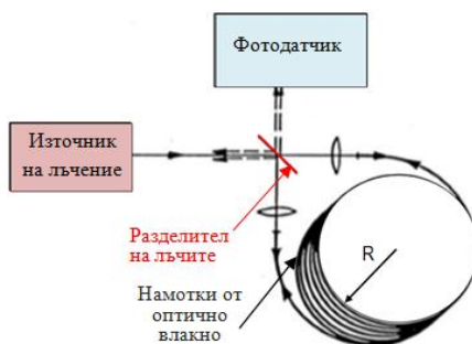
Фигура 14. Схема и основни елементи в устройството на FOG: източник, фотодетектор, намотка от оптично влакно, разделител на лъчите (сплитер).
