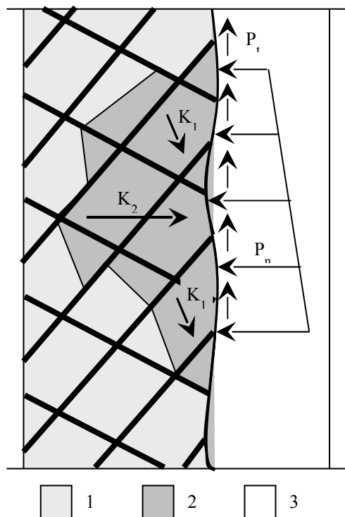
Фиг. 5. Взаимодействие между запълнението и страничните стени на добивното пространство с отчитане на структурната нарушеност на масива.
