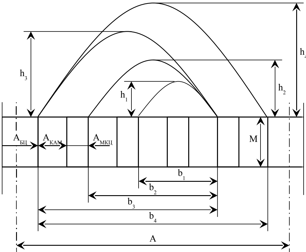
Фиг. 2. Параметри на камерно стълбова система на разработване и зони на обрушаване при разрушаване на междукamerни целици
