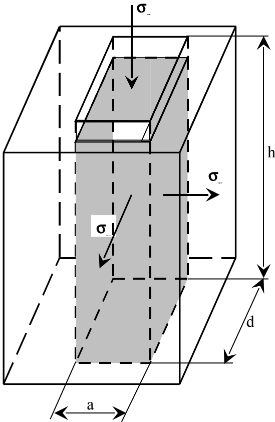
Фиг.3. Схема на съвместната работа на междукамерния целик и запълнението
