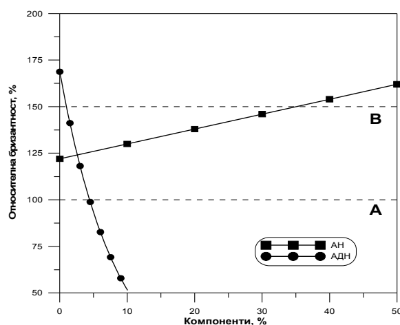
фиг.1. Зависимост на относителната бризантност от компонентите във взривни матрици от АН и АДН
