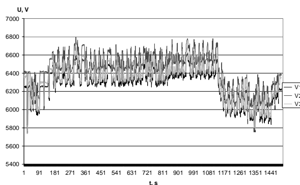
Фиг. 6. Напрежения на двигателя на багер Hitachi №10 при различни напрежения от подстанцията
