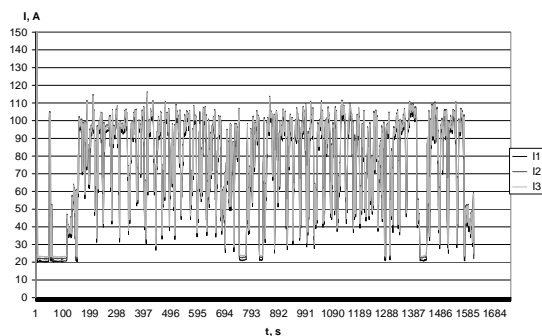
Фиг. 4. Фазни токове на багер №13
