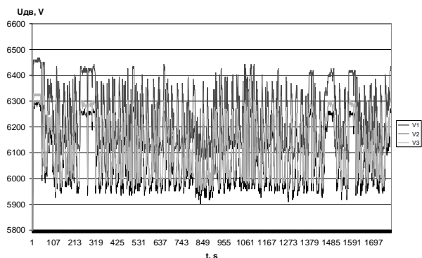
Фиг. 1. Напрежения на багер №10
