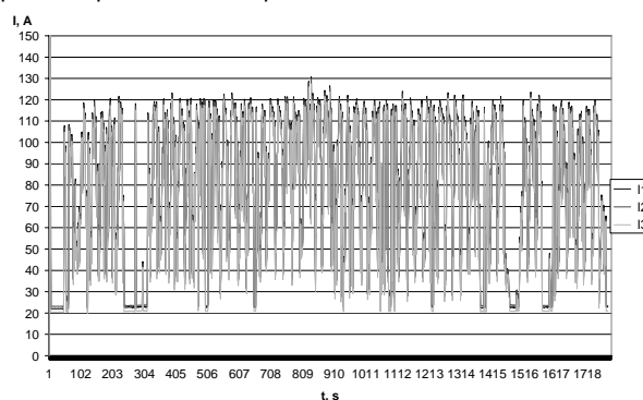
Фиг. 2. Фазни токове на багер №10
