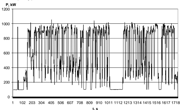
Фиг. 9. Консумирана от мрежата мощност на двигател на Hitachi №13
