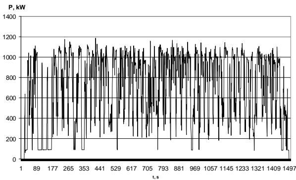
Фиг. 8. Консумирана от мрежата мощност на двигател на Hitachi №10
