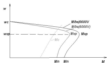
Фиг. 5. Механична характеристика на двигателя при различни захранващи напрежения
