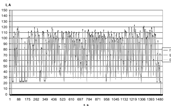
Фиг. 7. Изменение на фазните токове на двигателя на багер № 10 при промяна на напрежението
