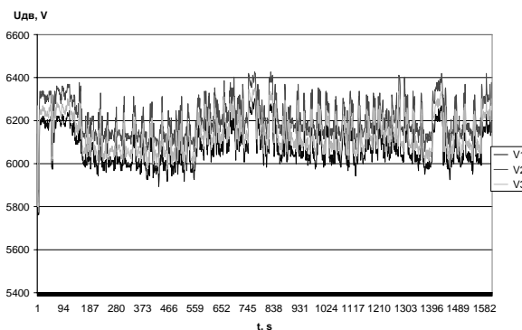
Фиг. 3. Напрежения на багер №13
