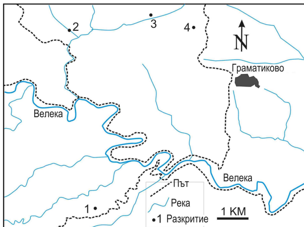
Фиг. 1. Находищата на диабаз с реликтови сферолити от ЮИ Странджа: 1 – Каменска бърчина; 2 – Малкораевски дол; 3 – Котвенски дол; 4 – река Стръвница
