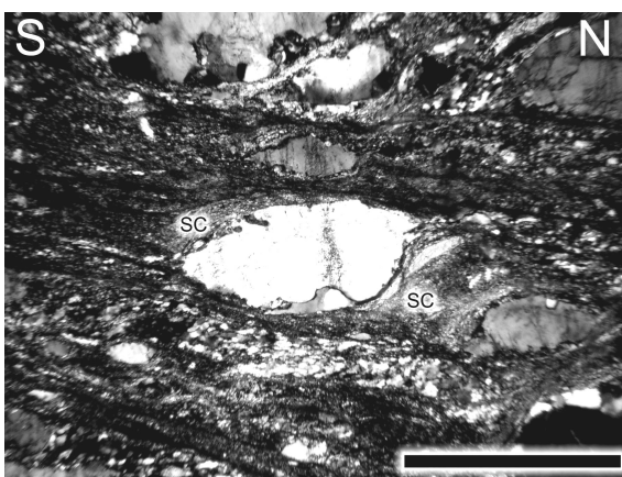
Фиг. 3. Асиметрични "опашки" и деформационни шапки (strain camps – sc), които заедно с ивици на сръзване индикатират насочени на север сръзвания. Мащаб 1 mm
