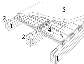
Фиг. 13 Изпълнение на подова конструкция от лепени греди, керамика и стоманобетон: 1) лепени греди от ламели; 2) монтажна арматура (поддържа арматурната мрежа на "работно" ниво във височина); 3) плоски тухли; 4) арматурна мрежа от \angle 6 [mm]; 5) тънка бетонна плоча;
