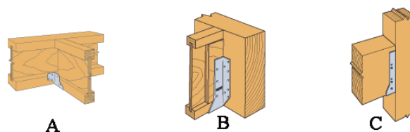
Фиг.3 Връзки - МН НУ НУС между дървени елементи от конструкцията: А – между Л”Т”ДГ с МН; В – между Л”Т”ДГ и ПДГ с НУ; С – между ребро и дървена колона (стойка) с НУС;
