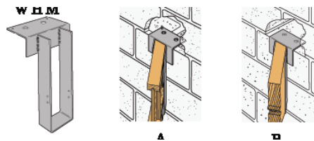
Фиг.6 Връзката WHM и нейното използване за монтаж на дървени гредови елементи под ъгъл: А – лепена двойно "Т" греда; В - ребро;
