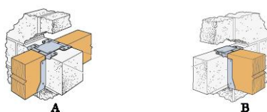
Фиг.5 Подпиране на греда към зидария: А – начин на подпиране на прекъснатата ПДГ от стена иззидана от газобетон посредством опорно устройство JHMS; В – подпиране на ПДГ в газобетонна стена чрез опорно устройство JHMR;
