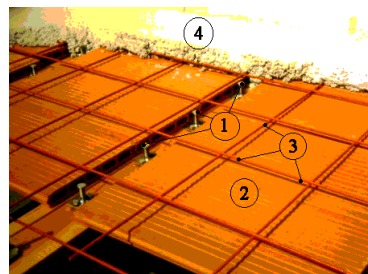
Фиг.15 Дървени греди с монтирани връзки (стоманени дюбели) - етап от изливане на плочата: 1) връзки между гредата и армираната плоча; 2) плоска тухла; 3) арматурна мрежа от \angle 6 mm; 4) тънка бетонна плоча;
