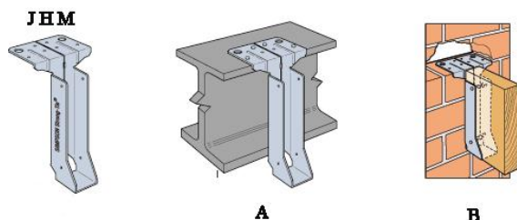
Фиг.4 Опорно устройство JHM и възли: А - между дървено ребро и стоманена двойно "Т" греда чрез JHM; В – същото устройство, предава натоварването от реброто на зидана стена;
