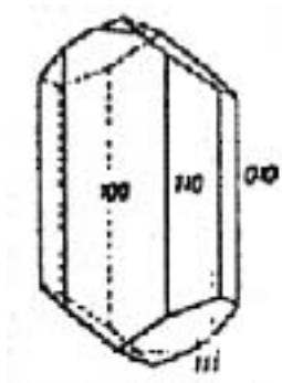
Фиг.86. Кристална форма на авгит
