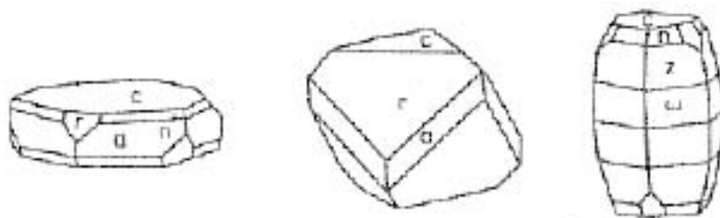
Фиг. 65. Кристални форми на корунд: c\{0001\} ; r\{10\bar{4}1\} ; n\{22\bar{4}3\} ; z\{22\bar{4}1\} ; w\{11\bar{2}1\} .
