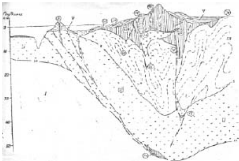
Фиг. 45. Схематичен разрез на земната кора под океаните (отляво) и под континентите ( по Роненсон ,1982) I - подкоров ; II - гранулитно - базалтов ; III - гранито - гнайсов ; IV - метаморфен ; V - седиментен ; граници : М на Мохорович ; К - на Конрад
