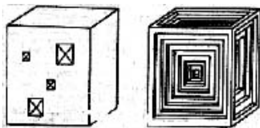
Кристална форма и скелетен кристал на халит
