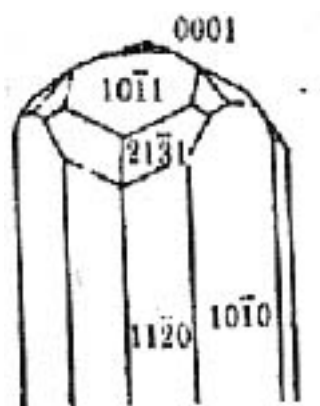
Фиг. 84. Кристална форма на турмалин
