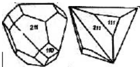
Фиг.60. Кристални форми на тетраедрит
