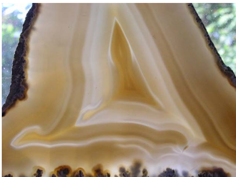
Ахат, Кърджалийско, колекция М. Токмачиева
