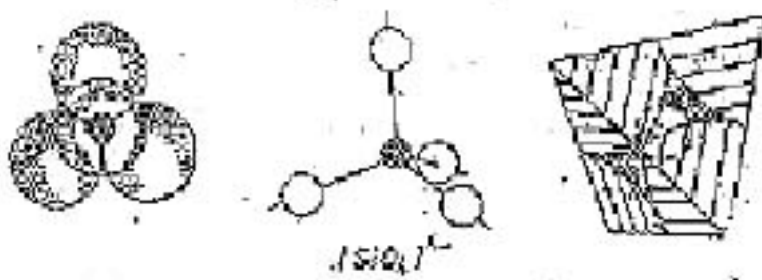
Фиг. 77. Силиций - кислородна тетраедрична група
