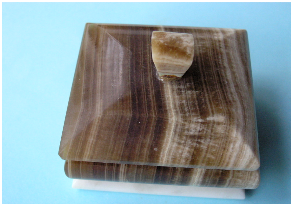
Арагонит (Изремец, Врачанско, изделие-Русия, колекция М. Токмачиева)
