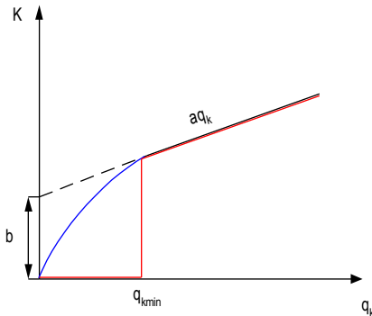
фиг. 1 Зависимост на капиталовложенията от мощността на к.б.
