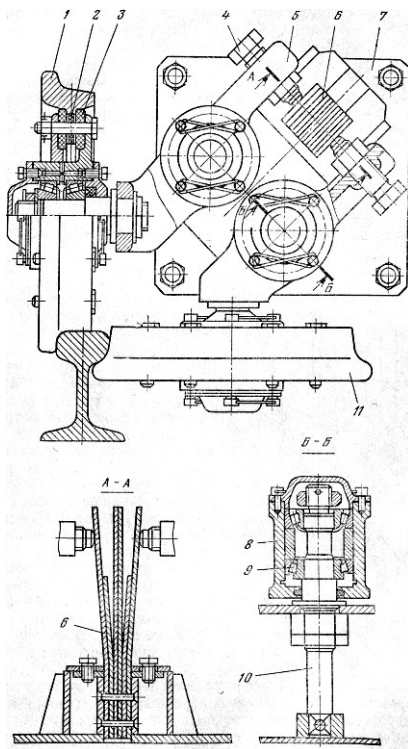
Фиг. 3. Двуколесен направляващ апарат за релсови водачи и едностранно водене на подемния съд:
