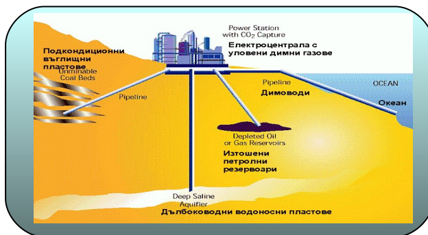
Фигура 2. Основни възможности за депониране на CO 2
