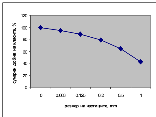
Фиг. 1. Зърнометрична характеристика на въглищата от мина "Черно море"
