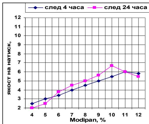
Фиг. 7. Зависимост между разхода на свързващо вещество Modipan и якостта на натиск на произведените брикети с въглища класа 6–0 mm., изследвана след съответно 4 и 24 часов престой на брикетите
