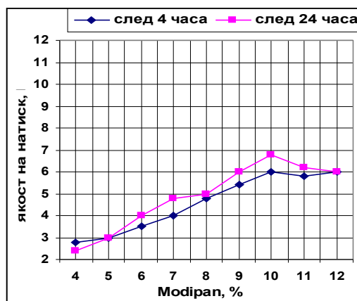
Фиг. 6. Зависимост между разхода на свързващо вещество Modipan и якостта на натиск на произведените брикети с въглища класа 4-0 mm., изследвана след съответно 4 и 24 часов престой на брикетите
