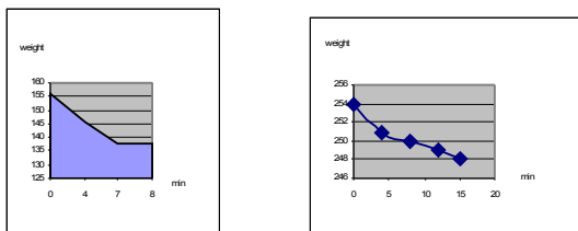
а/ б/ Фиг. 4. Кинетика на смилане, а/ обкатаване на тела с овална форма, б/ обкатаване на тела с „лоша“ форма.
