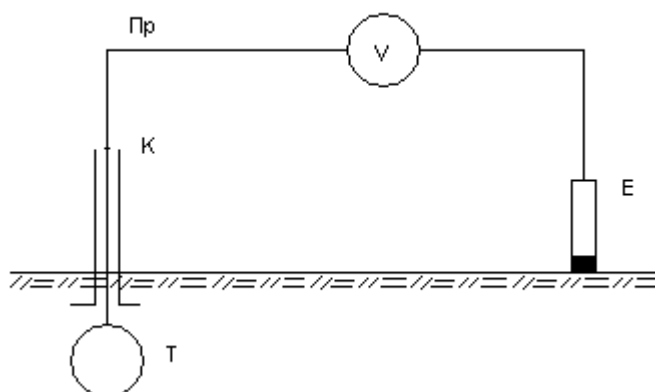
фиг. 1. схема за измерване на потенциалната разлика "съоръжение-земя"
