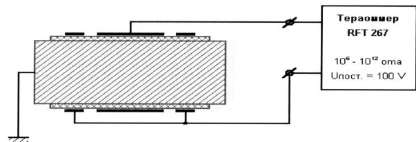
Фиг. 5. Опитна постановка за измерване на специфичното повърхностно съпротивление
