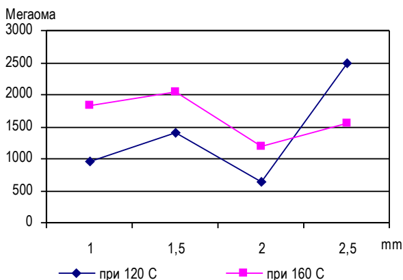
Фиг.7. Специфично повърхностно съпротивление при различни дебелини на изолацията
