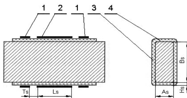
Фиг. 2. Подготовка на образца за измерване на специфичното обемно съпротивление
