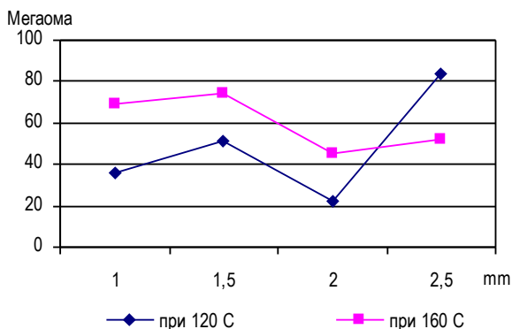
Фиг. 6. Измерено повърхностно съпротивление при различни дебелини на изолацията
