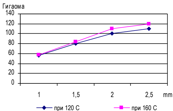
Фиг. 3. Измерено обемно съпротивление при различна дебелина на изолацията
