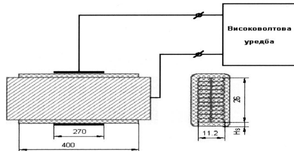
Фиг. 8. Опитна постановка за изчисляване на обемния и повърхностен ток през изолацията
