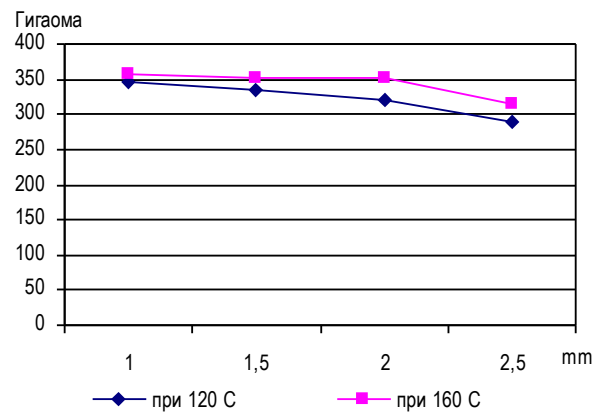
Фиг. 4. Специфично обемно съпротивление при различни дебелини на изолацията
