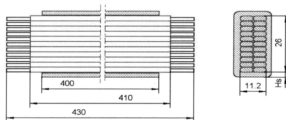
Фиг. 1. Размери на опитния образец
