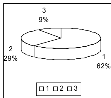
Фигура 8. Разход на труд (в %) за изпълнение на стенен елемент по МН, с размери: височина 350cm, широчина 150 cm и дебелина: а) d=18 cm; б) d=30 cm; в) d=40 cm.
