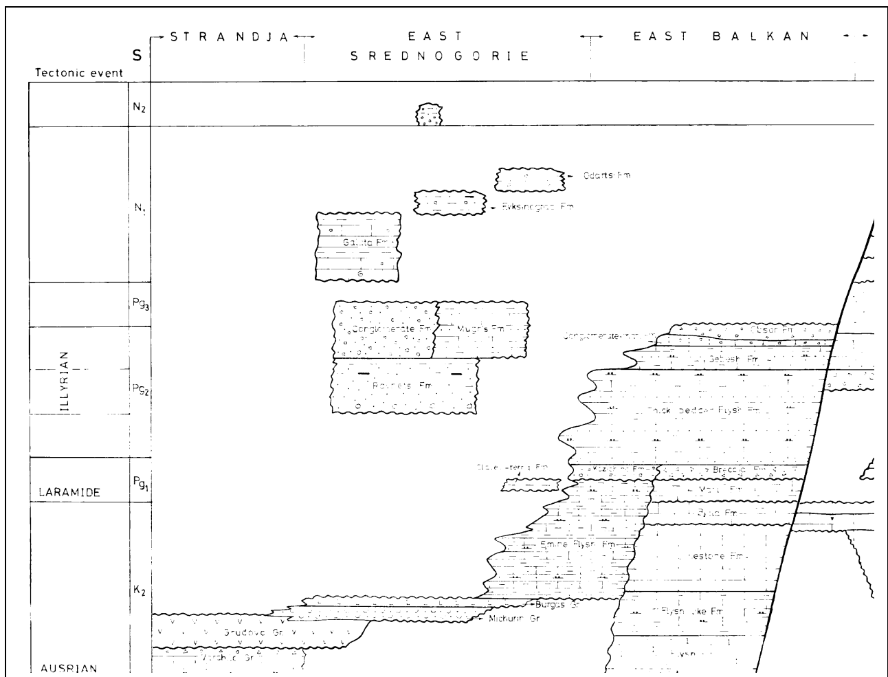
Фиг. 2. Литостратиграфска подябла на терциерните седименти в Югоизточна България (по данни от геоложкото картиране)
