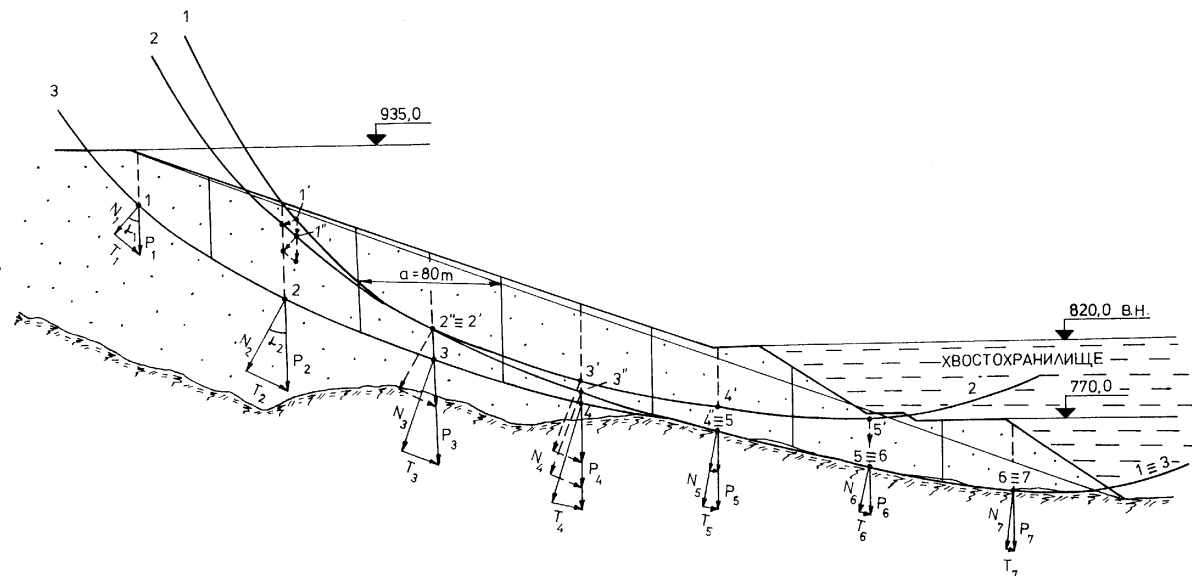
Фиг. 2. Изчисляване устойчивостта на откоса на Западното насипище на хор. 935 по профил 10-10
