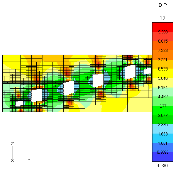
Фиг. 56. Стойности на коефициента на устойчивост Drucker-Prager (вертикална равнина)
