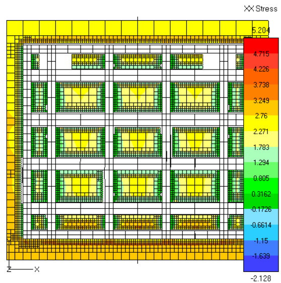
Фиг. 8а. Горизонтални напрежения \sigma_{xx}
