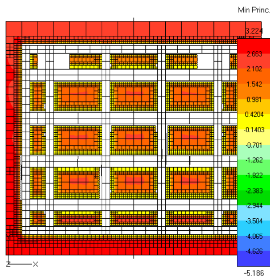
Фиг. 4а. Минимално главно напрежение
