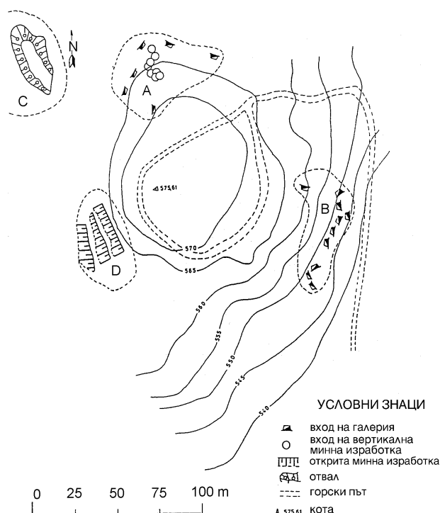
Фигура 3. Схема за разположението на входовете на минните изработки : А.) шахти; Б.) галерии; В.) отвали с отбит материал; Г.) кариера за открит добив
