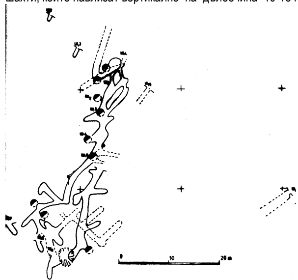
Фигура 5. План на минните изработки (шахти, галерии и комини) в северозападната част на хълма Хисар Тепе
