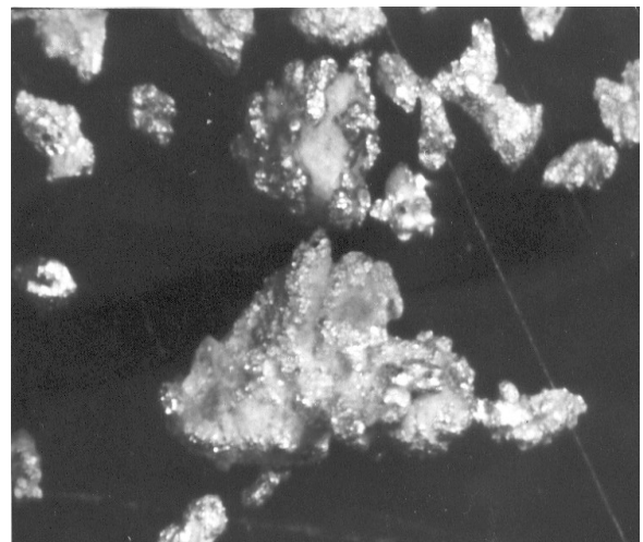
Фигура 9. Микрофотография на златни зърна, извлечени от почвения слой на хълма Хисар Тепе. Увел.100x
