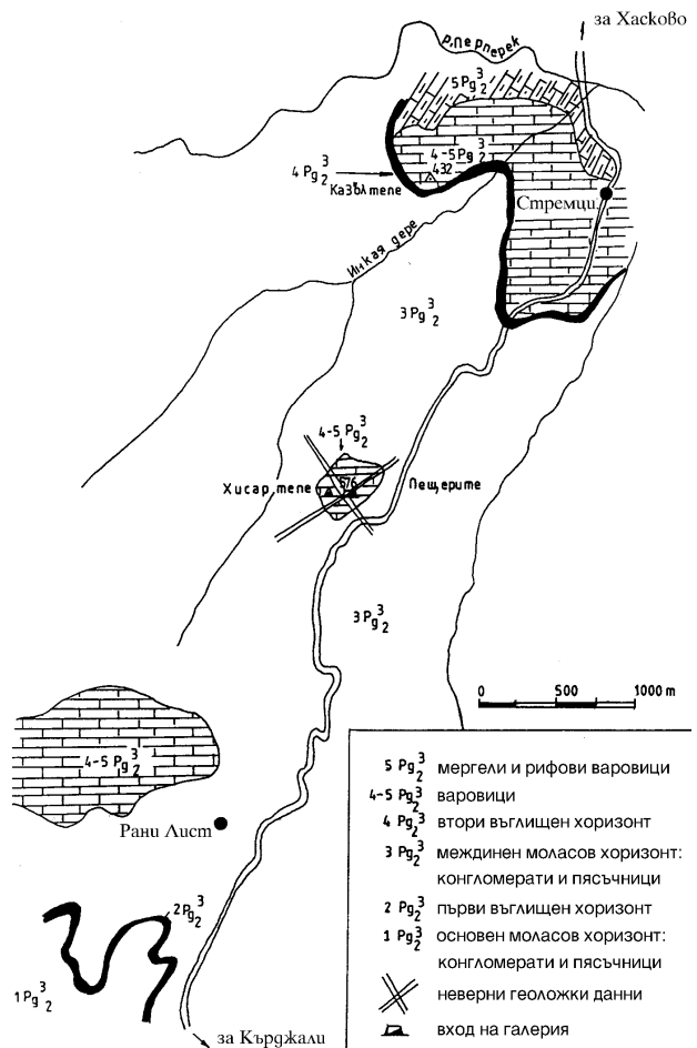
Фигура 2. Геоложка карта на района по Д. Минчев и др.; 1963, с допълнения от автора
